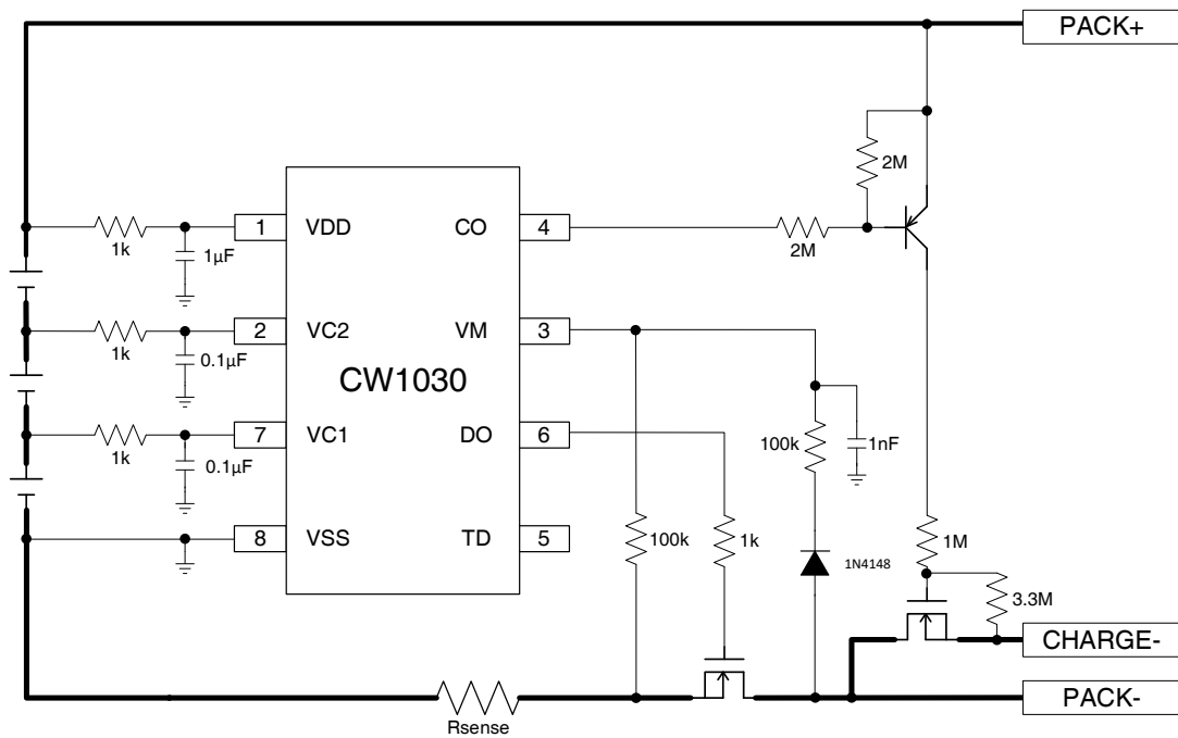
带采样电阻应用电路
