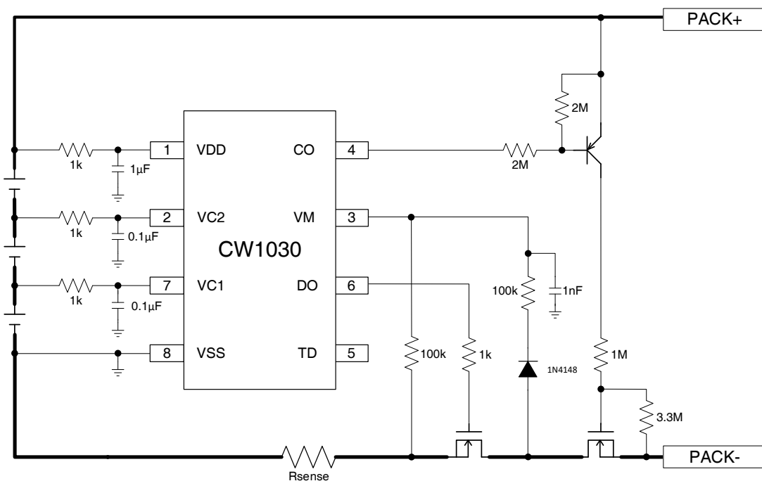
带采样电阻同口应用电路
