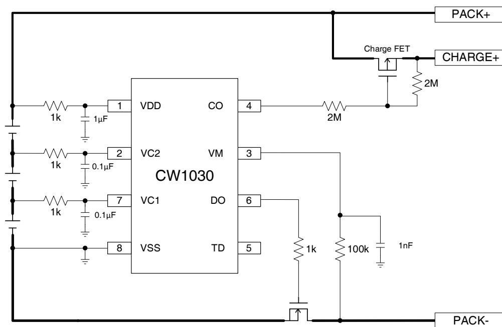
3 串共负异口应用电路
