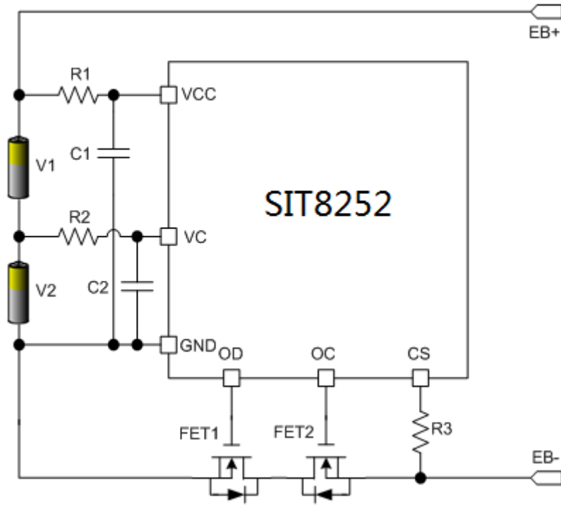
图 6. SIT8252 典型应用电路
