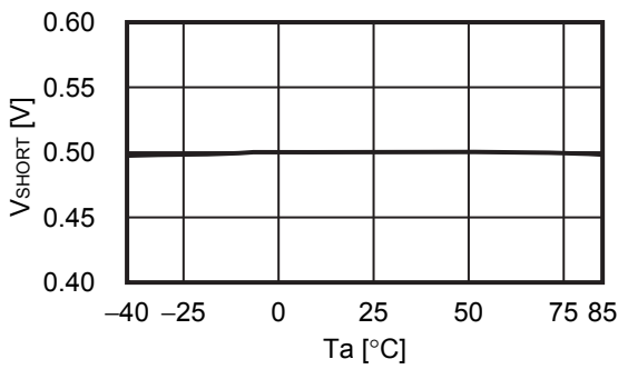
2.13 V_{\text{SH ORT}} - T_a
