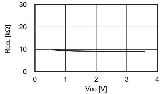
3.4 R_{DOL} - V_{DO}
