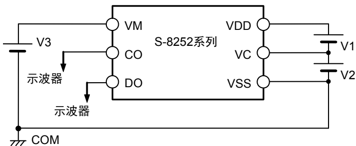
图9 测定电路5
